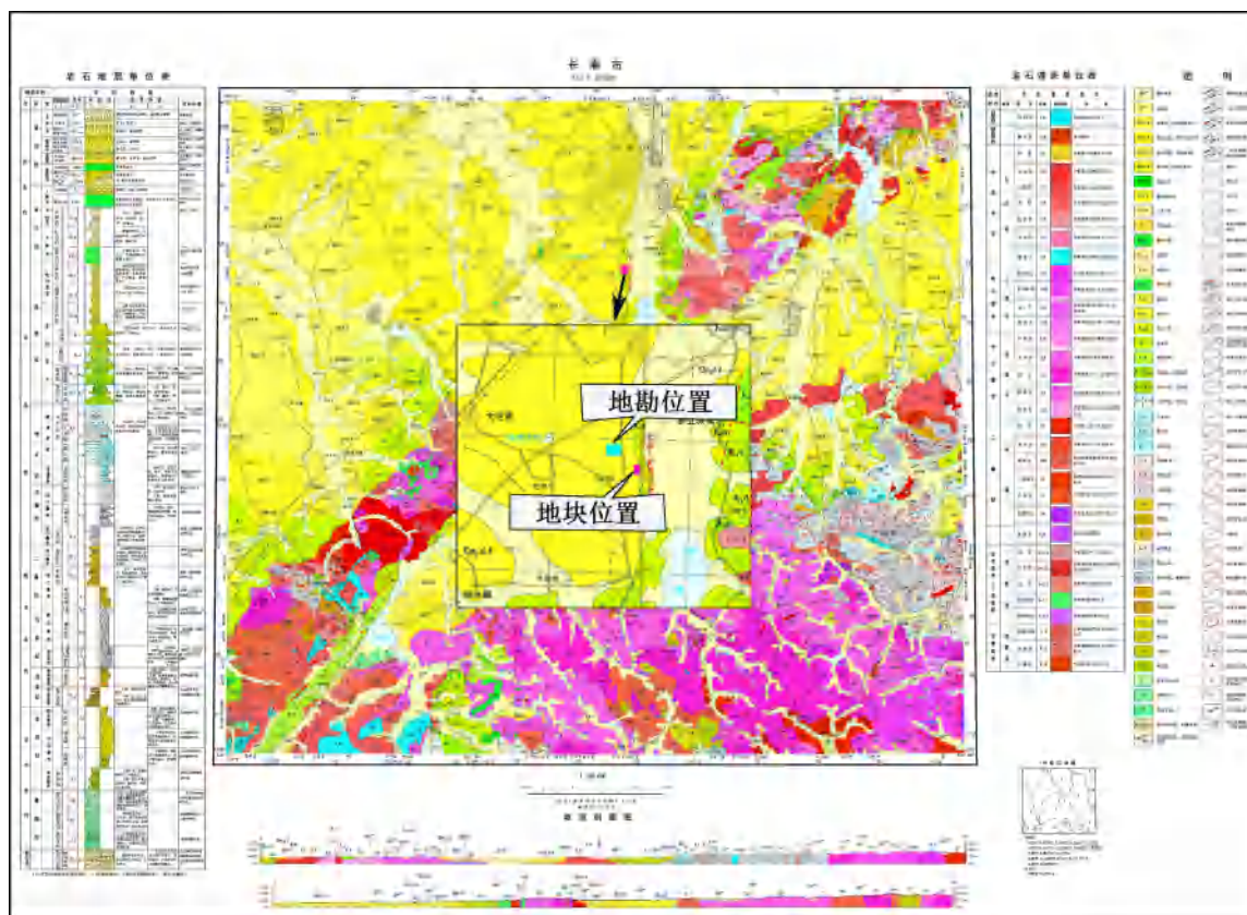
图 5-1 区域地质图
